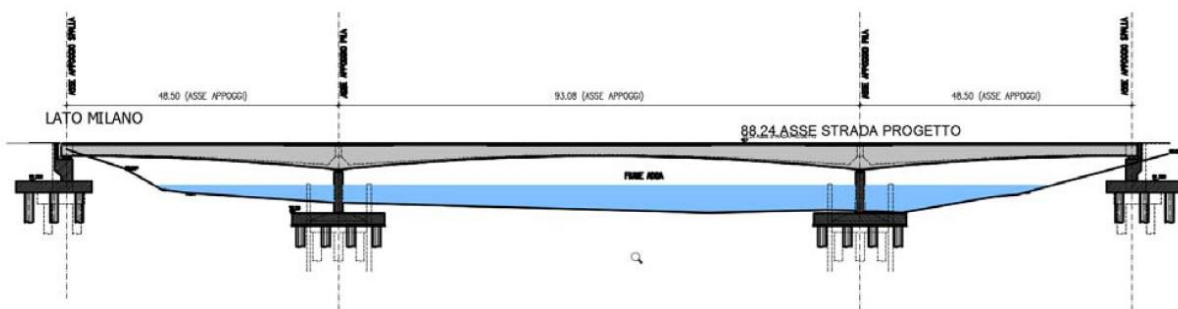
Prospetto del nuovo ponte sull'Adda che consentirà il raddoppio della sezione stradale
